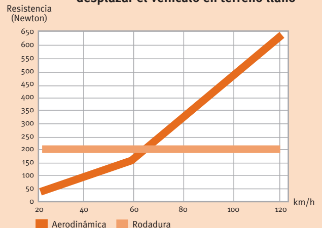
Resistencias que ha de vencer el motor para desplazar el vehículo en terreno llano
